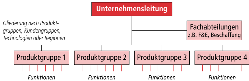
Abbildung 3.13: Divisionale Organisation
